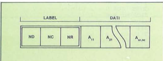
Figura 3 - Formato di immagazzinamento delle matrici su dischetto. Vanno ordinate per colonne, facendo precedere ai dati una label con le seguenti informazioni: ND = sempre uguale a 2 (numero delle dimensioni) - NC = numero delle colonne - NR = numero delle righe.
